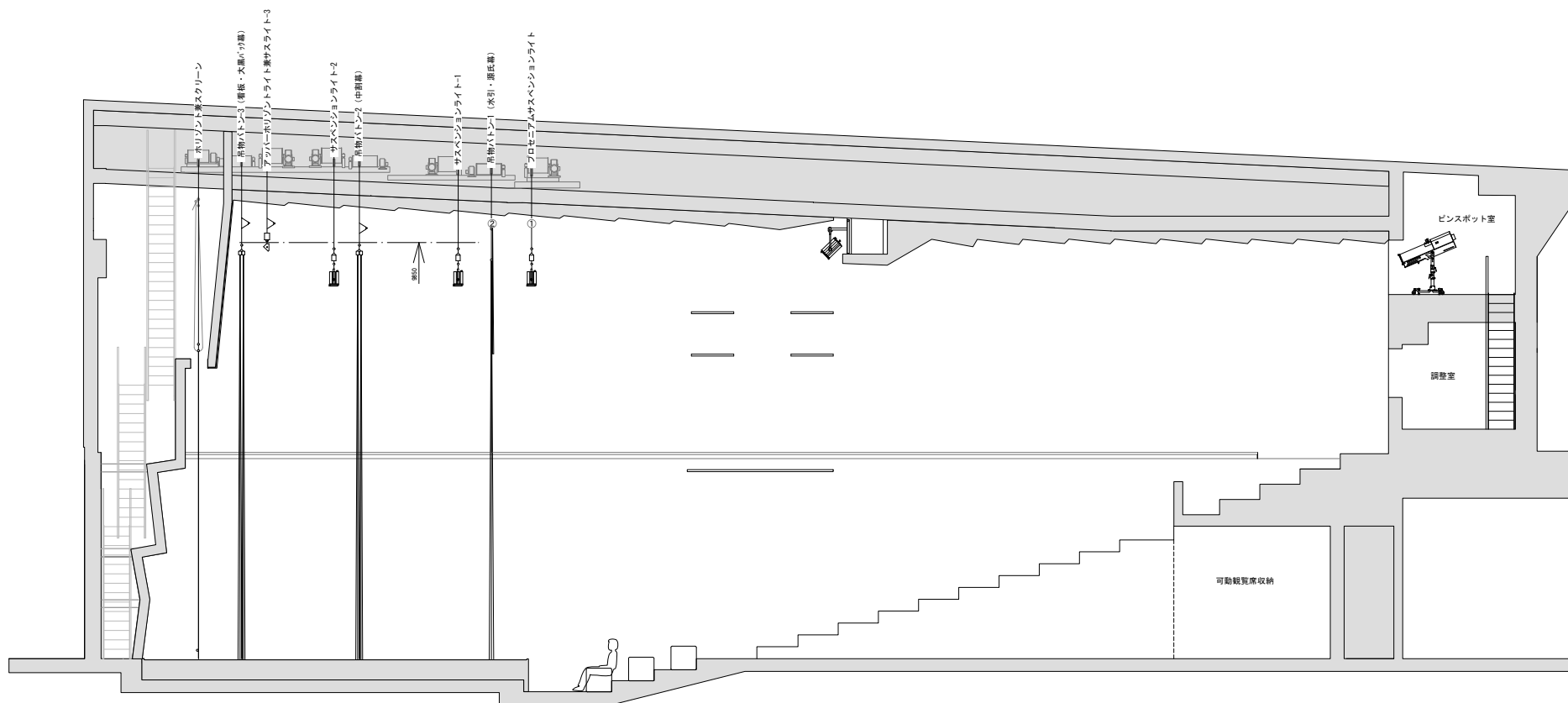
舞台断面図 (S=1/75)
